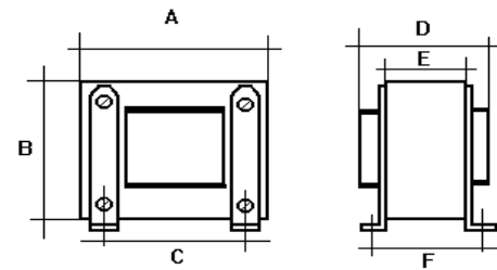
Fig 2 Dimensiones físicas
