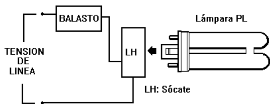
Fig. 1 Diagrama esquemático de conexión
