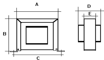
Fig 2 Dimensiones físicas
